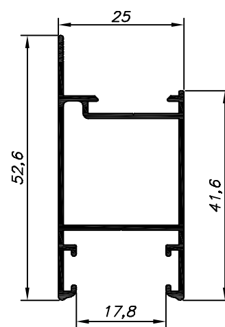
SU-039 2.840 Kg/Barra 6m 2.180 Kg/Barra 4,6m
