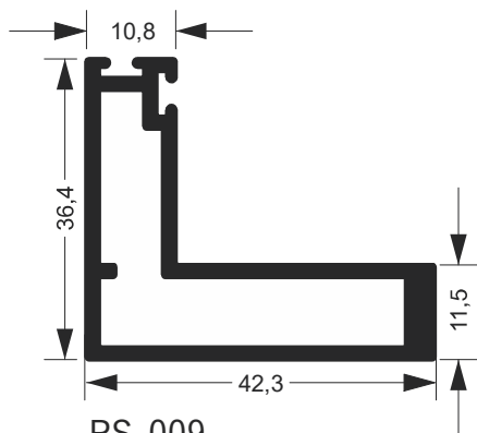
PS-009 4.567Kg/Barra 6m
